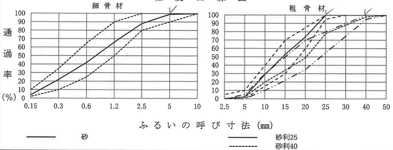
粒度曲線図
