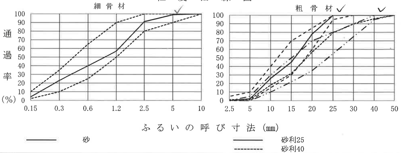
粒 度 曲 線 図
