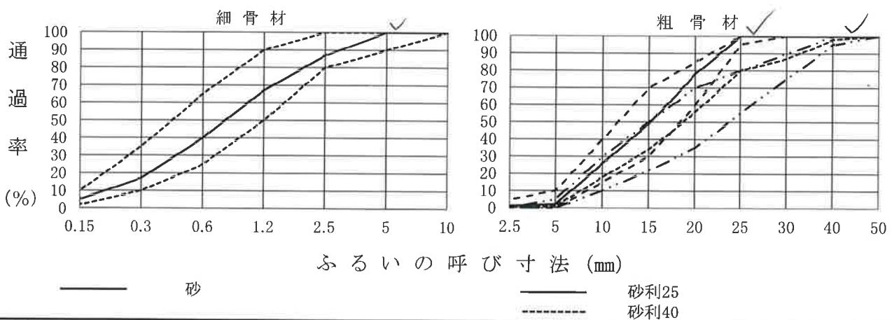
粒 度 曲 線 図
