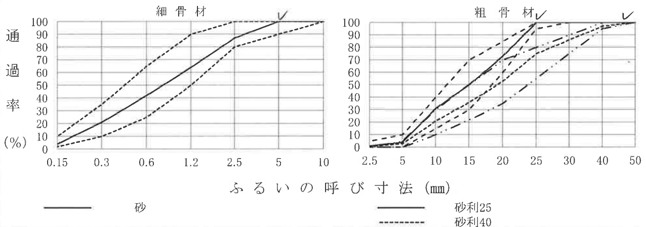
粒 度 曲 線 図
