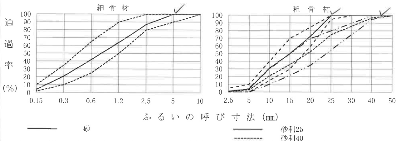
粒 度 曲 線 図
