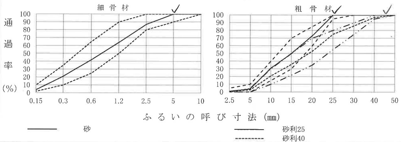
粒 度 曲 線 図
