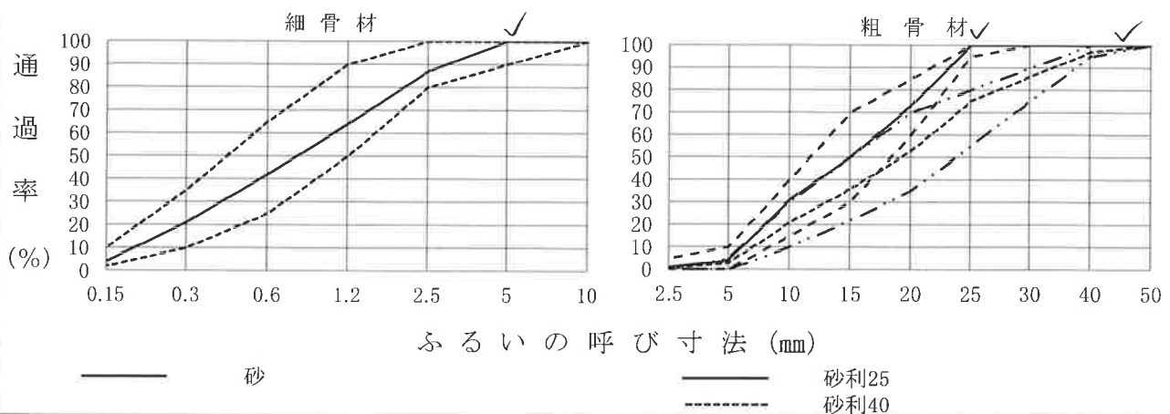
粒 度 曲 線 図
