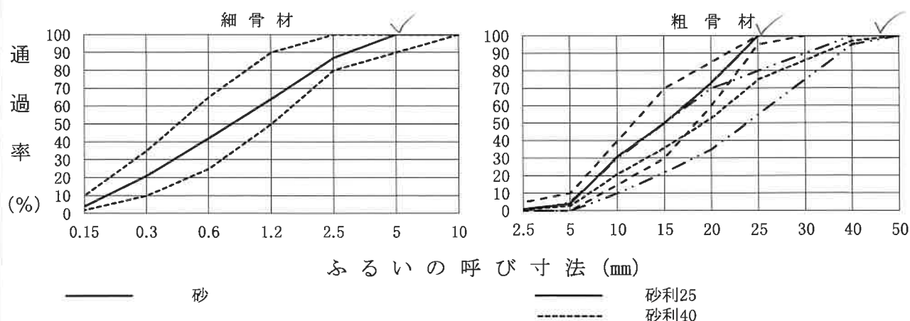
粒 度 曲 線 図
