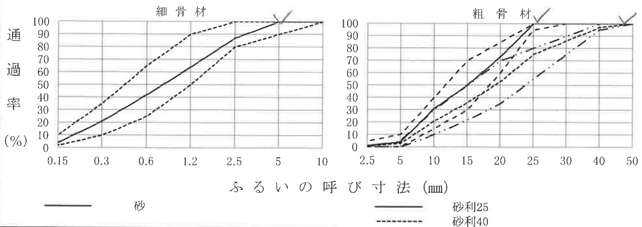
粒 度 曲 線 図
